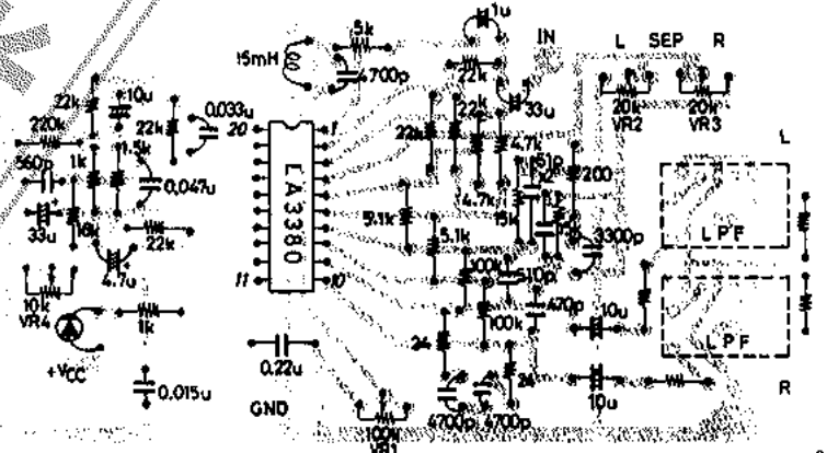
プリントパターン例 (銅箔面)
